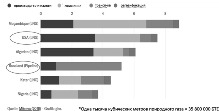
Рис. 9. Стоимость (издержки) поставок природного газа (сжиженного – LNG и трубопроводного – Pipeline) в Европу, в долл. на миллион британских тепловых единиц (БТЕ)*
